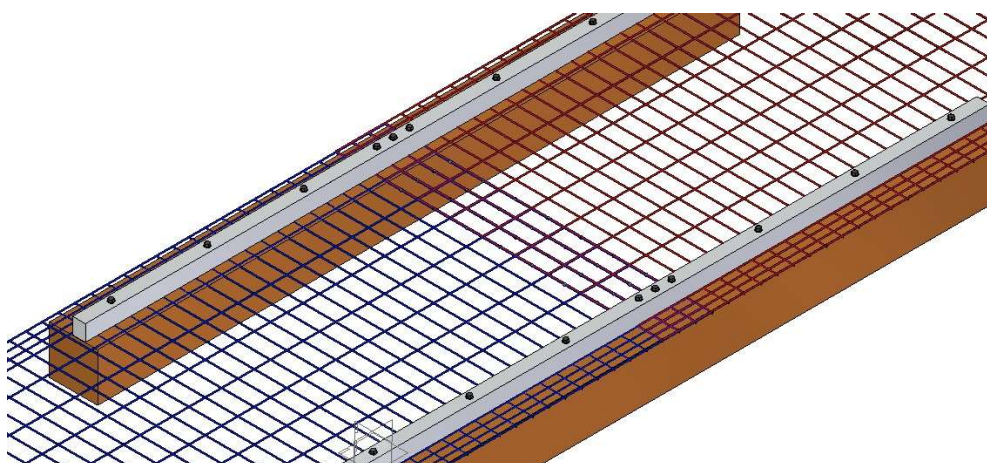
Giunzione fra rotoli con gancetti ad anello - un elemento di fissaggio per ogni maglia sovrapposta
