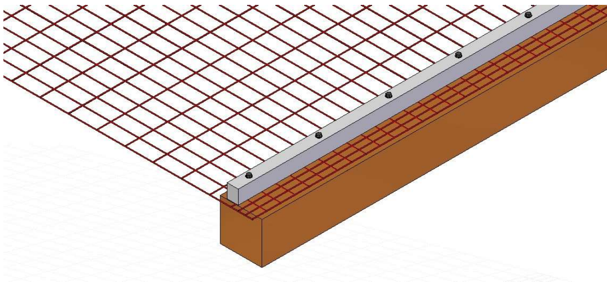
Rete con giunzione longitudinale - Fissaggi passo 25 cm
