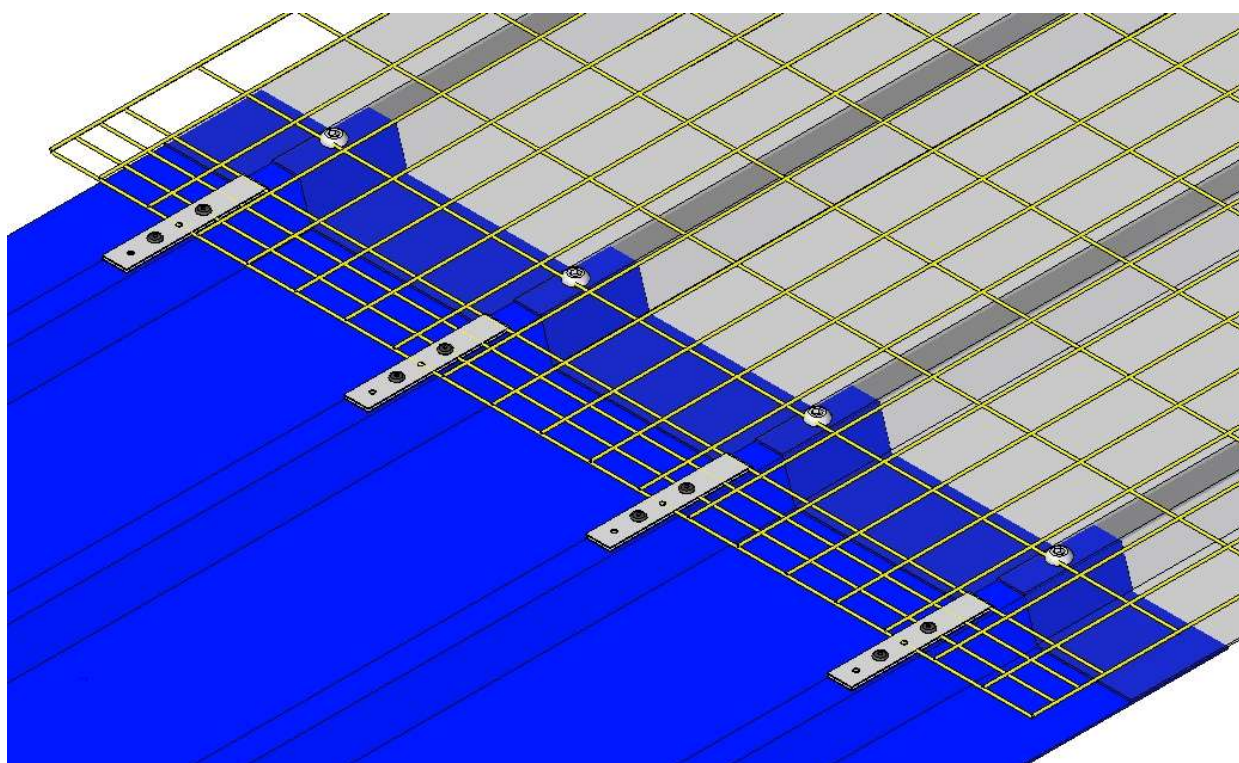
Rete anticaduta su lamiera grecata e lucernario in polycarbonato in sormonto
