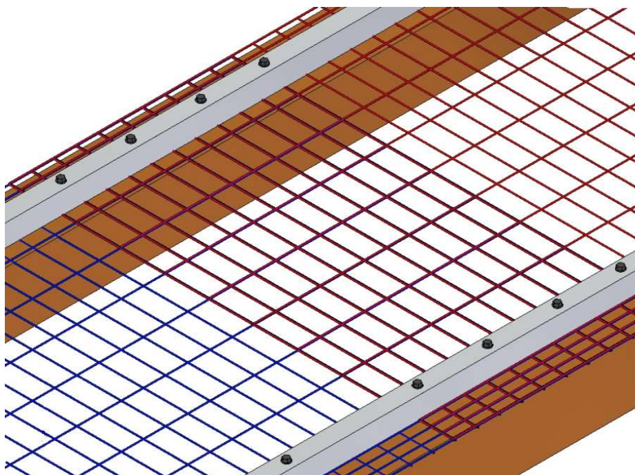
Giunzione fra rotoli senza gancetti ad anello - elementi di fissaggio a passo dimezzato
