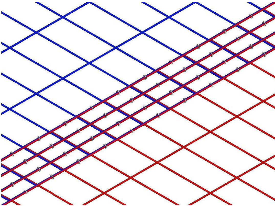
Rete con giunzione longitudinale - Giunzione con sovrapposizione dei 4 fili di cimosa e fissaggio con gancetti ad anello
