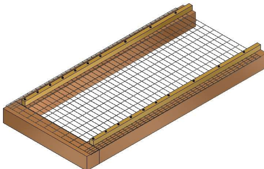
Fissaggio della rete senza elemento di ancoraggio in testata
