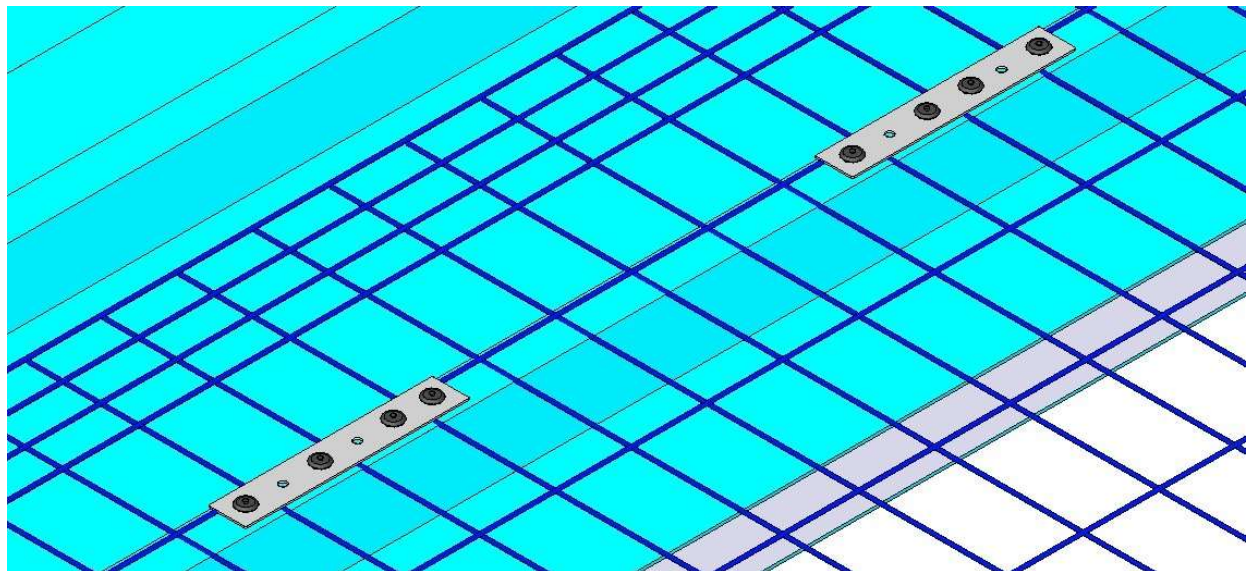
Rete anticaduta su pannello grecato - Rete perpendicolare al profilo grecato Larghezza del lucernario ridotta - 4 rivetti per piastrina
