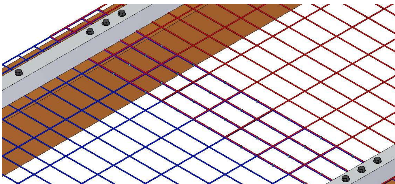
Giunzione fra rotoli con gancetti ad anello - gancetti su 3 maglie - 4 fili
