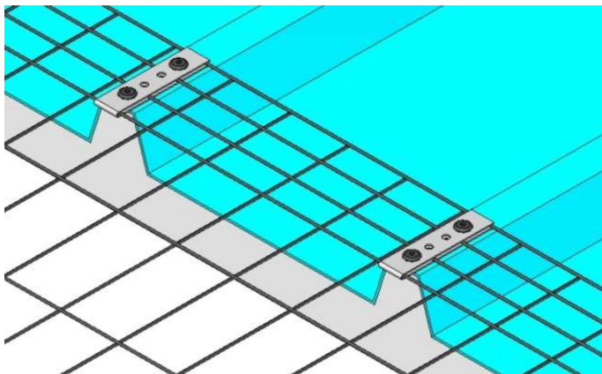
Rete anticaduta su pannello grecato - Rete parallela al profilo grecato
