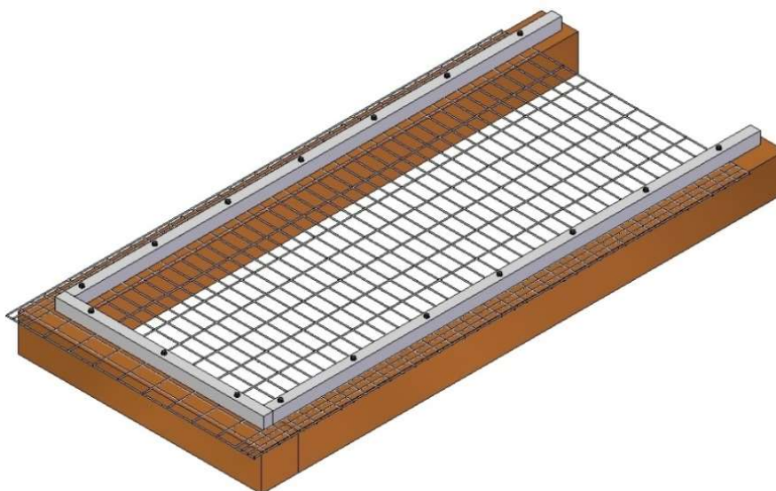
Fissaggio della rete con lo stesso elemento di ancoraggio in testata
