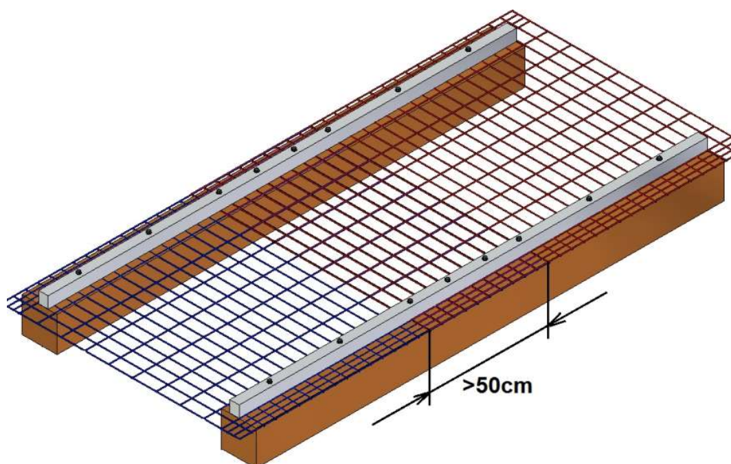
Giunzione fra rotoli senza gancetti ad anello - elementi di fissaggio a passo dimezzato
