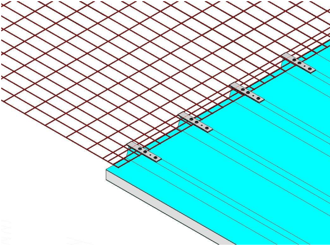
Rete con giunzione longitudinale - Fissaggi passo 25 cm
