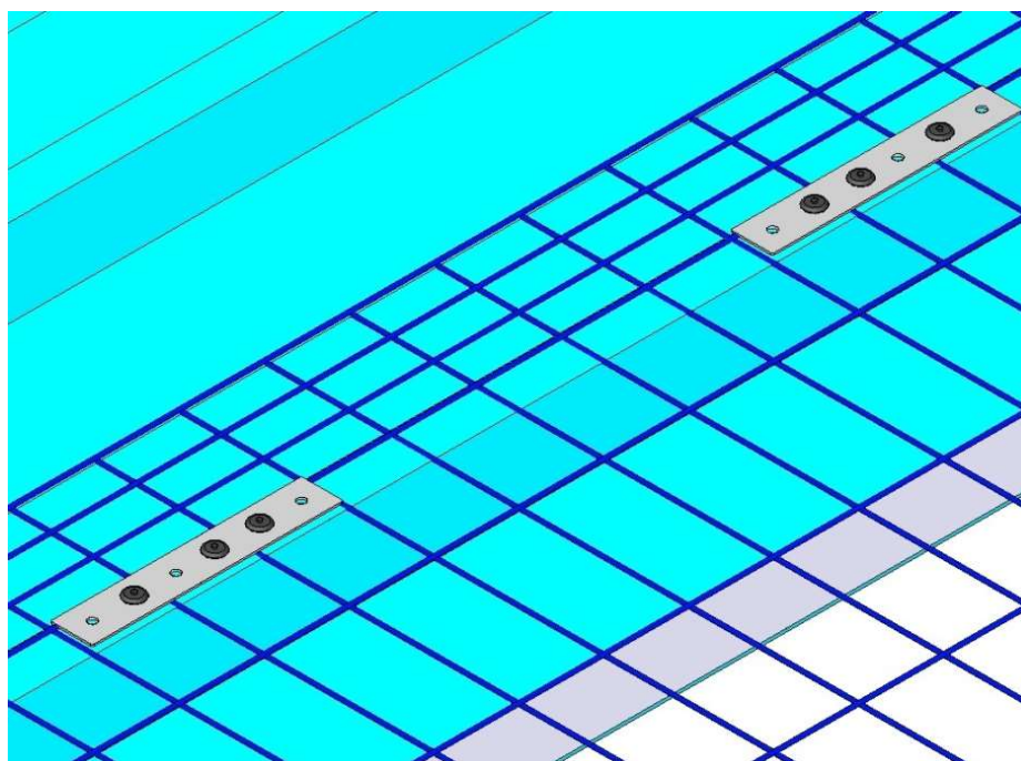
Rete anticaduta su pannello grecato - Rete perpendicolare al profilo grecato
